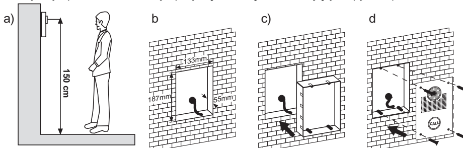
Rys 9. Montaż panela zewnętrznego
