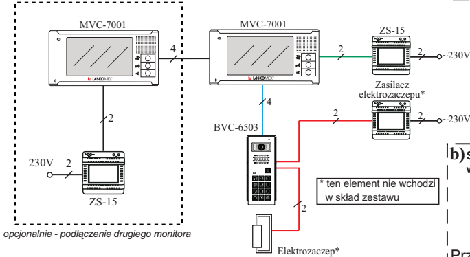
Rys 4. Podłączenie zestawu wideodomofonowego Apus - schemat jednokreskowy
