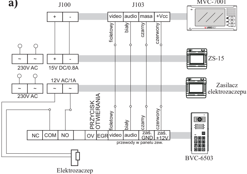
Rys 5. a) Schemat podłączenia elementów zestawu wideodomofonowego Apus.
