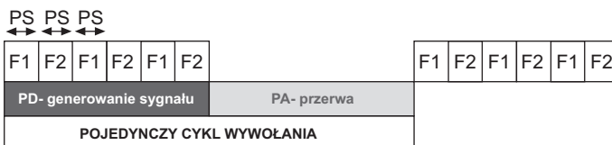
Rys. 8.1 Struktura sygnału wywołania
