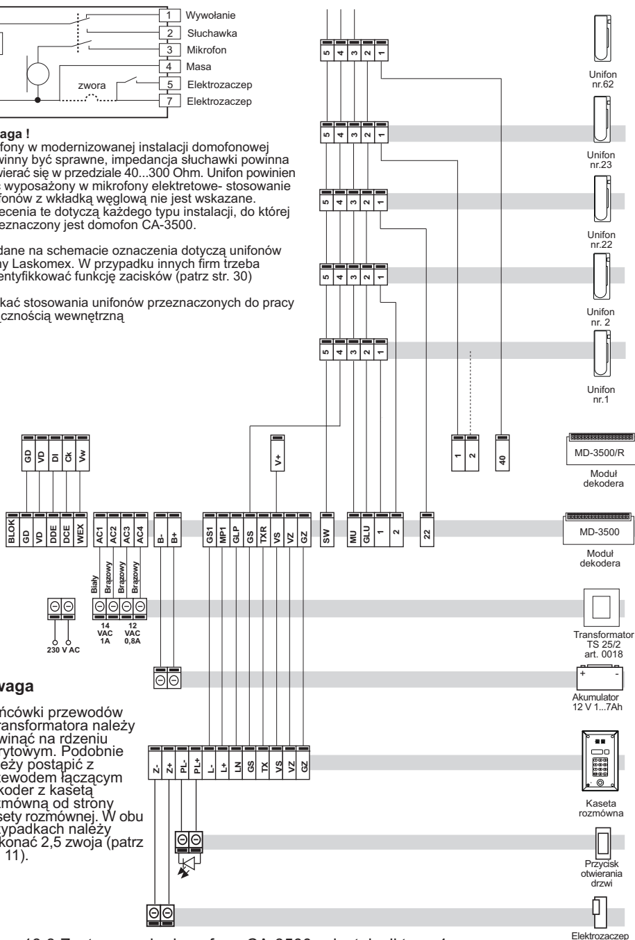
Rys. 13.3 Zastosowanie domofonu CA-3500 w instalacji typu 4+n
